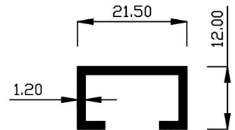
11409 0.151Kg/m
