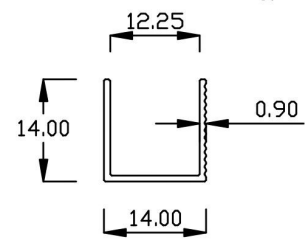
17570 0.590Kg/m
