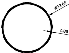
17569 0.162Kg/m
