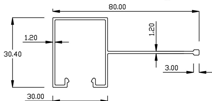
17570 0.590Kg/m
