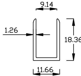
17570 0.590Kg/m
