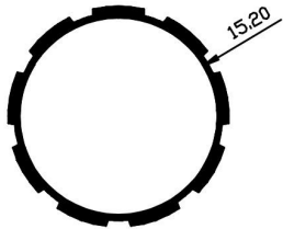
12303 0.276 Kg/m
