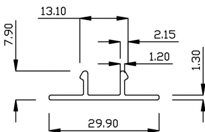
17569 0.162Kg/m
