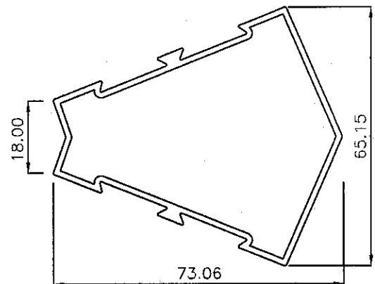
12278 0.978Kg/m
